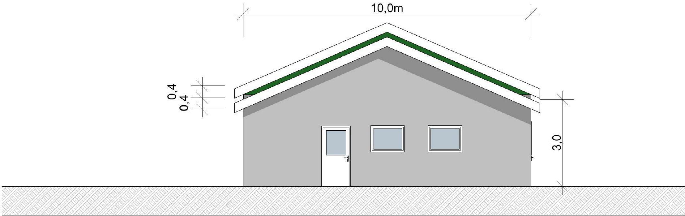
1:100 Fasade nord-vest
